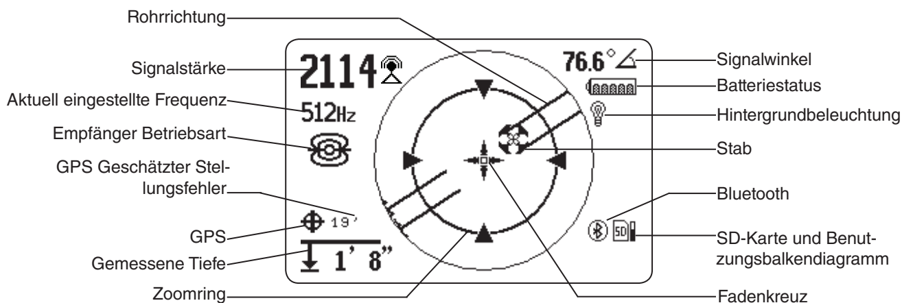
Abbildung 2 – Sondenmodus-Anzeige, Beispiel
